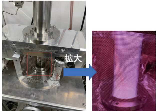
図4: カーボンニュートラル検討用プラズマ合成基本装置
